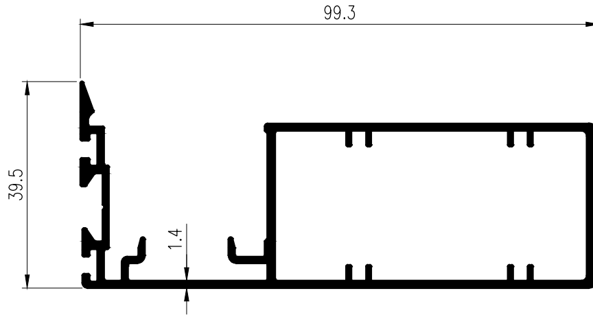
T-15667 WT : 1.281 kg./m.
