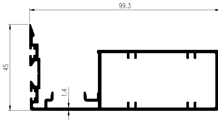
T-15777 WT : 1.320 kg./m.
