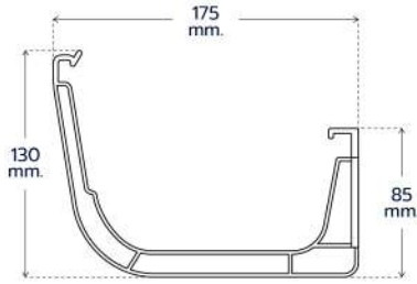
STANDARD BRACKET ตะขอรับราง
