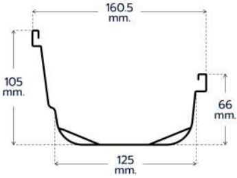
GUTTER รางน้ำฝน
