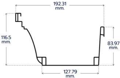
GUTTER รางน้ำฝน
