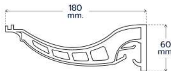
INVISIBLE HANGER ตะขอแขวนราง
