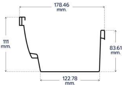
GUTTER รางน้ำฝน
