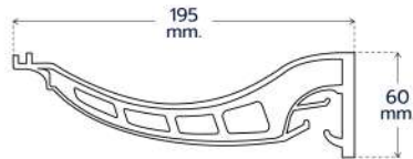
INVISIBLE HANGER ตะขอแขวนราง
