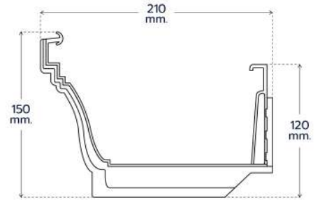
STANDARD BRACKET ตะขอรับราง
