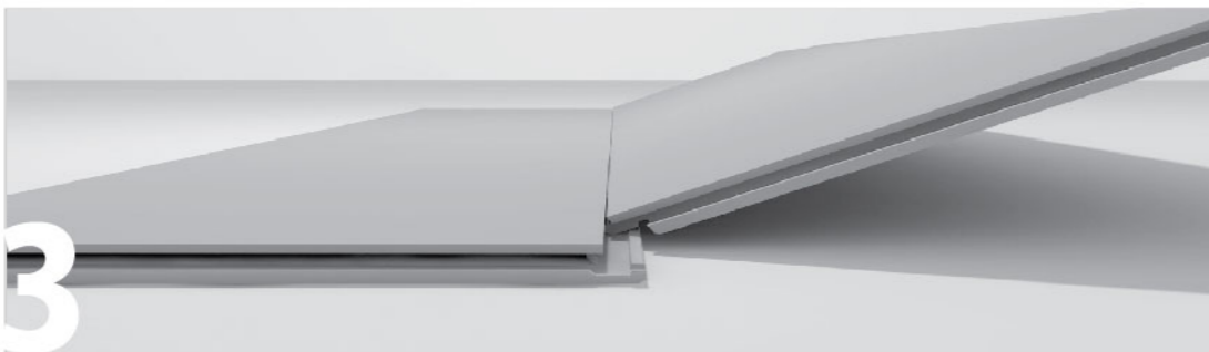
3 การวางพื้นไวนิลต่อกันให้หันด้านร่อง และด้านเติงเข้าหากันโดยทำมุมเอียง 45 องศา With 45 degree angle tilt embedded
