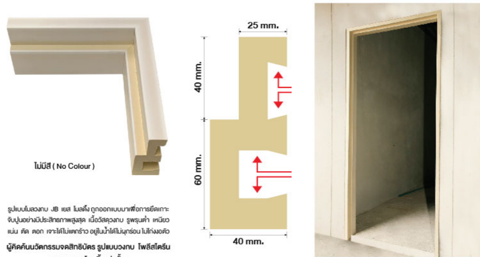
วงกบประตูรุ่น JB ระบบการติดตั้งแบบเปียก 1 ชุด มาพร้อมกับ เหล็กฉาก และเหล็กยึด
