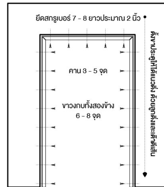
ติดชั๊วงกบกับงานใน ชั้นตอนสุดท้าย
