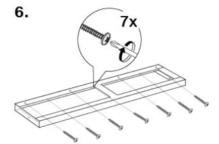
6. ยึดสกรูกับโครงเหล็ก ตามตำแหน่งพุก
